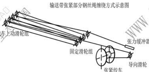
张紧绞车
