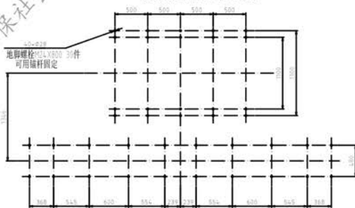
机头地脚螺栓平面布置图
